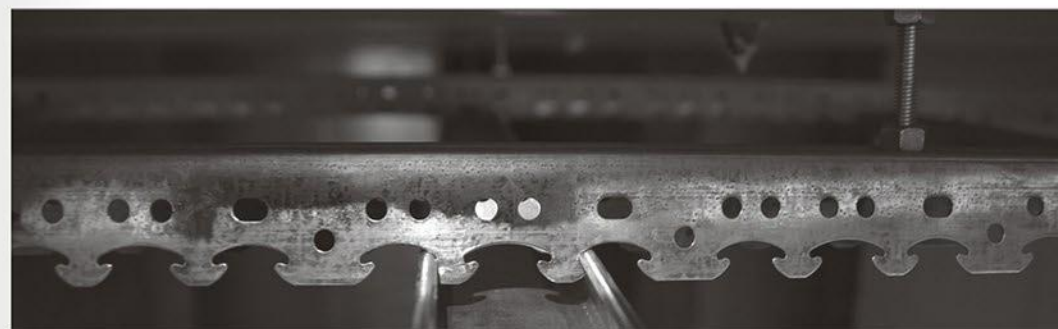
与 60 副龙骨配合
