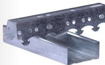
与 60 副龙骨配合
