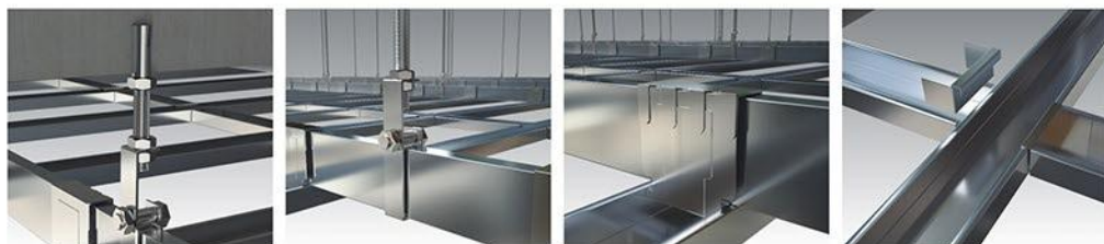
吊杆与天花板的连接点 主吊、吊杆、主骨的连接点 挂件与主骨及副骨之间的连接 水平件应用的连接
